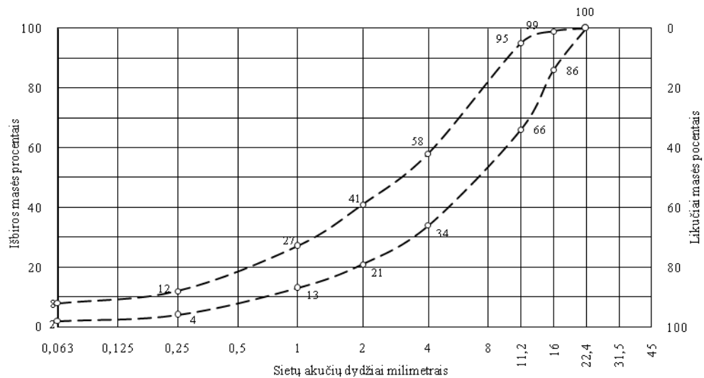
2 pav. Asfalto viršutinio sluoksnio mišinys SA 16-d tipas C
