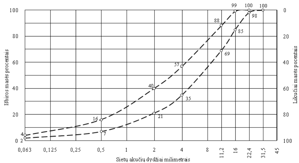
4 pav. Asfalto viršutinio sluoksnio asfaltbetonio mišinys SA 16-o tipas S
