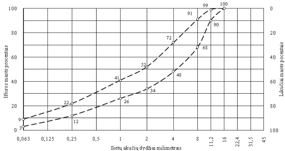
3 pav. Asfalto viršutinio sluoksnio asfaltbetonio mišinys SA 11-d tipas C
