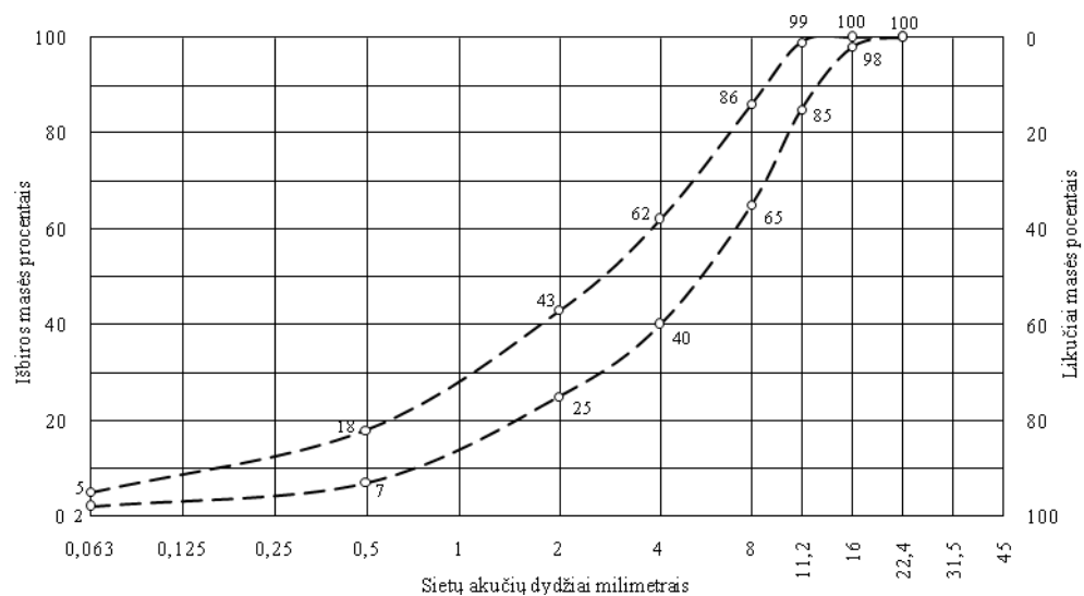
5 pav. Asfalto viršutinio sluoksnio asfaltbetonio mišinys SA 11-o tipas S
