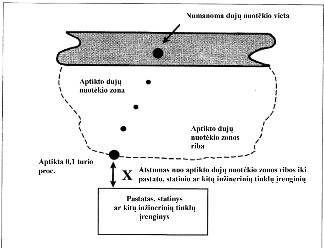
1 paveikslas. Dujų nuotėkio vietos klasės nustatymo pavyzdys
